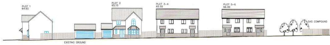
SECTION A-A
